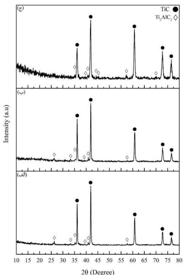
شکل ۳- الگوهای پراش پرتو ایکس مربوط به سیستم‌های ترکیبی: (الف) 2TiC-Al-Ti-0.1Si، (ب) 2TiC-Al-Ti-0.2Si و
