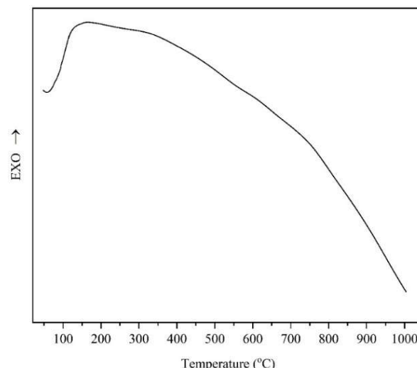
شکل ۲- منحنی گرماسنجی افتراقی سیستم ترکیبی
