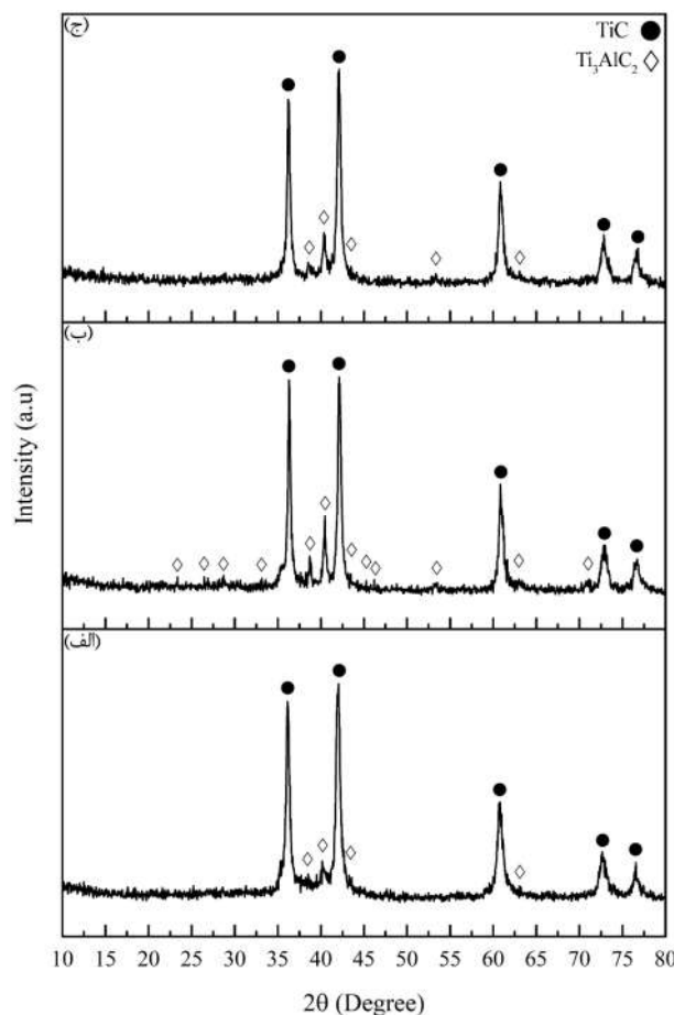
شکل ۱- الگوهای پراش پرتو ایکس مربوط به سیستم‌های ترکیبی: (الف) 2\text{TiC}-\text{Al}-\text{Ti}-0.1\text{Si} ، (ب) 2\text{TiC}-\text{Al}-\text{Ti}-0.2\text{Si} و (ج) 2\text{TiC}-\text{Al}-\text{Ti}-0.3\text{Si} پس از انجام فرایند آسیاب‌کاری به مدت ۲۵ ساعت.
