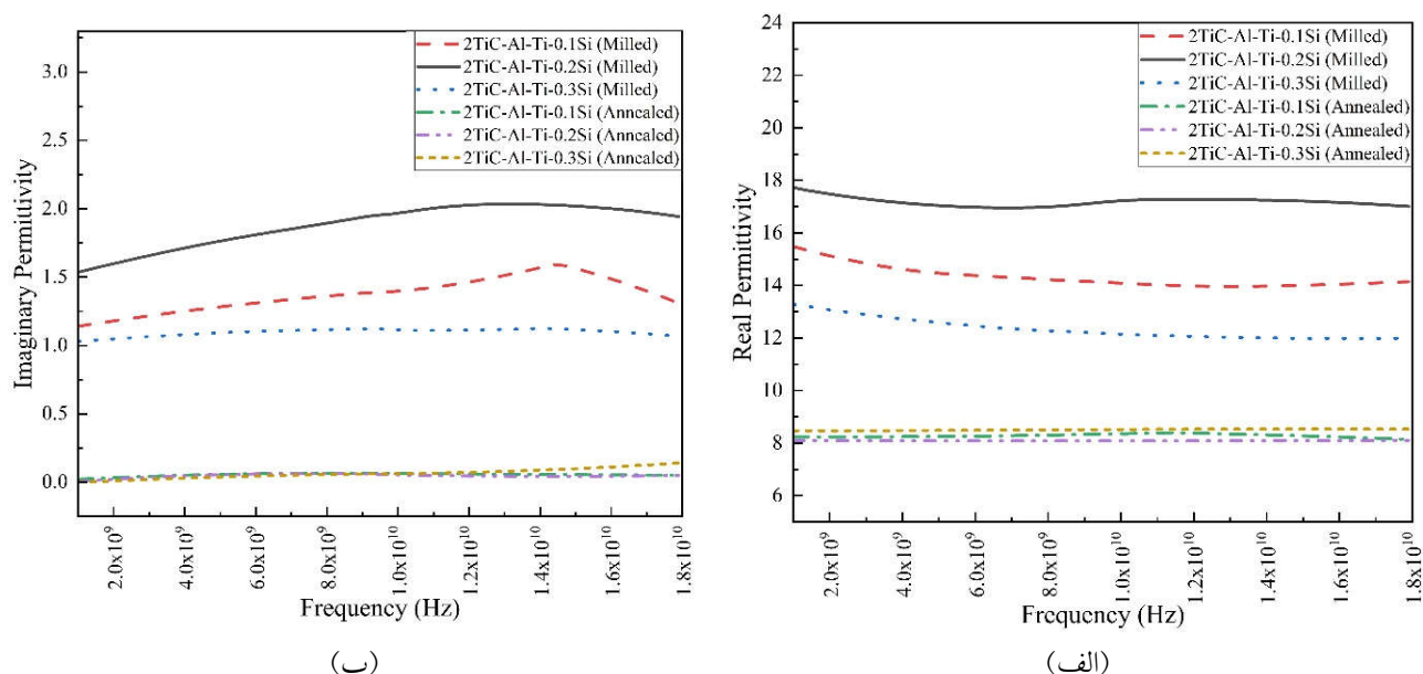
شکل ۶- نمودار گذردهی الکتریکی (الف) حقیقی ( \epsilon' )، (ب) موهومی ( \epsilon'' ) مربوط به سیستم‌های ترکیبی 2TiC-Al-Ti-xSi ( x=0.1, 0.2, 0.3 ) آسیاب‌شده و آنیل‌شده.
