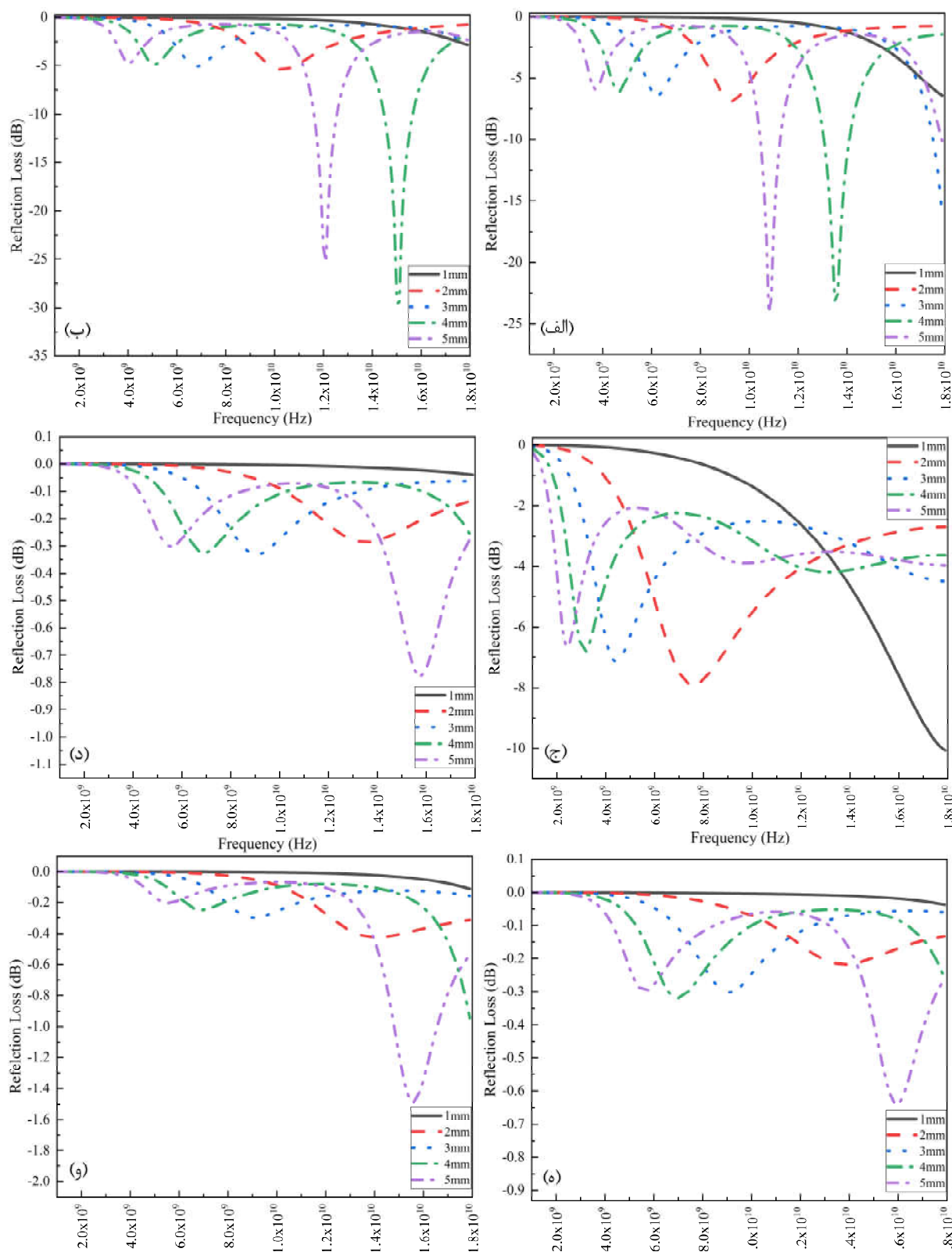
شکل ۷- نمودار تلفات انعکاس مربوط به سیستم‌های ترکیبی (الف) 2\text{TiC-Al-Ti-0.1Si} ، (ب) 2\text{TiC-Al-Ti-0.2Si} ، (ج) 2\text{TiC-Al-Ti-0.3Si} و سیستم‌های ترکیبی (د) 2\text{TiC-Al-Ti-0.1Si} ، (ه) 2\text{TiC-Al-Ti-0.2Si} و (و) 2\text{TiC-Al-Ti-0.3Si} آنیل شده در دمای 1400^\circ\text{C} درجه سانتی‌گراد به مدت ۵ ساعت.
