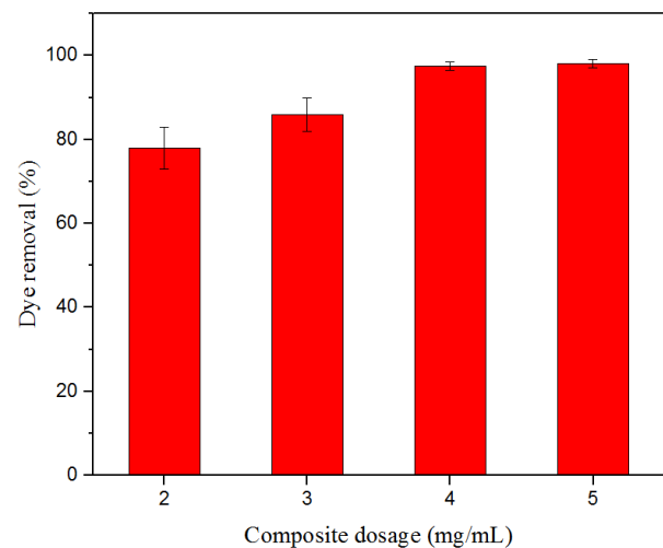
شکل ۸- جذب رنگ متیل اورانژ توسط کامپوزیت آلومینا-اکسید روی در وزن‌های مختلف.
