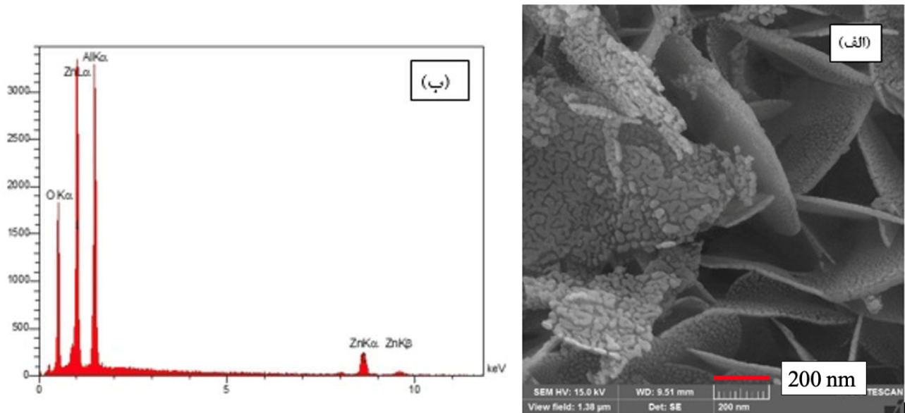
شکل ۳- الف) تصویر FE-SEM و ب) EDS، مربوط به نانوکامپوزیت آلومینا- اکسید روی کلسینه شده در دمای ۴۰۰ درجه سانتی‌گراد به مدت دو ساعت.
