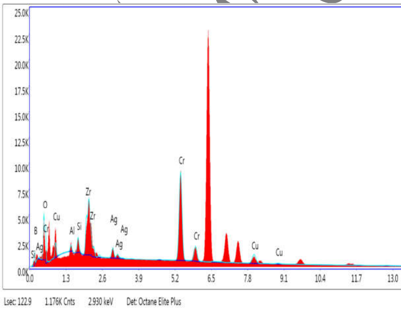
شکل ۴- نقشه توزیع عنصری و آنالیز شیمیایی عناصر آلیاژی مختلف موجود در ترکیب هدف تولید شده توسط دستگاه SPS.
