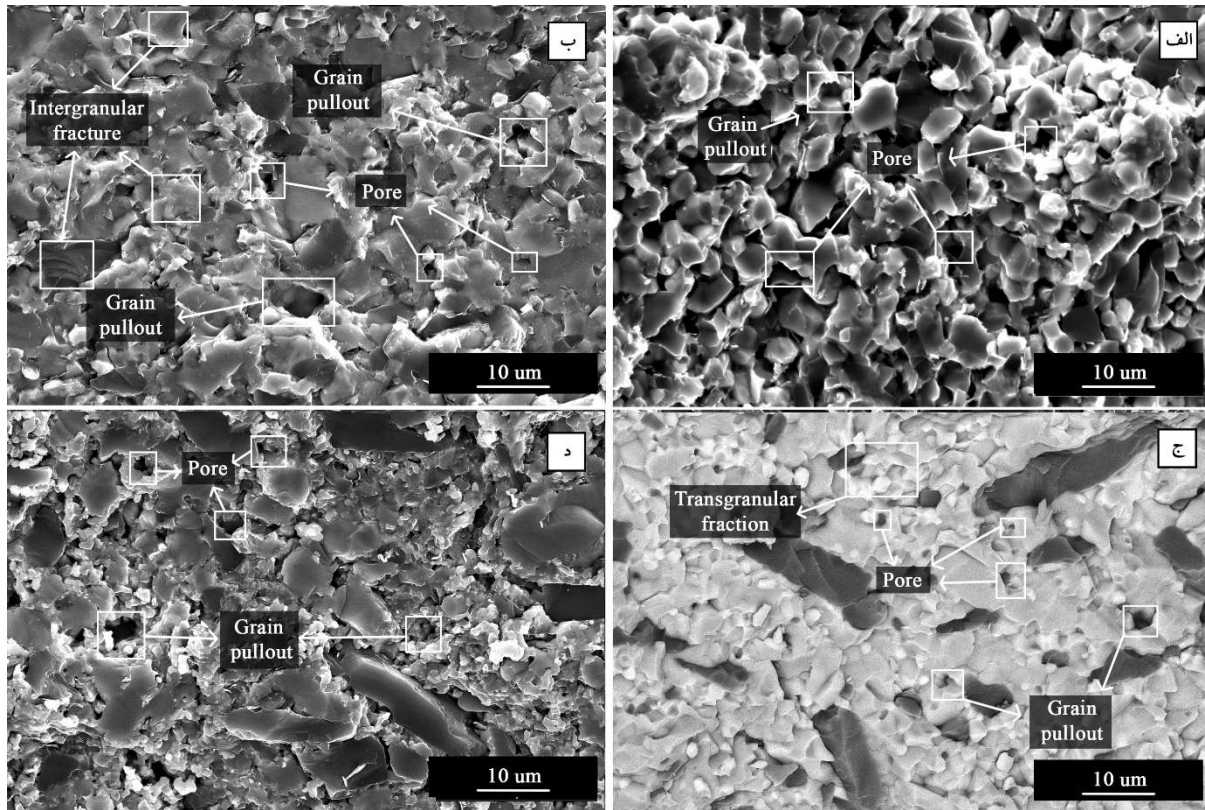
شکل ۵- تصویر FESEM از سطح شکست کامپوزیت (الف) ZS (ب) ZS5T (ج) ZS10T (د) ZS15T تفجوشی شده در دمای °C 1180.
