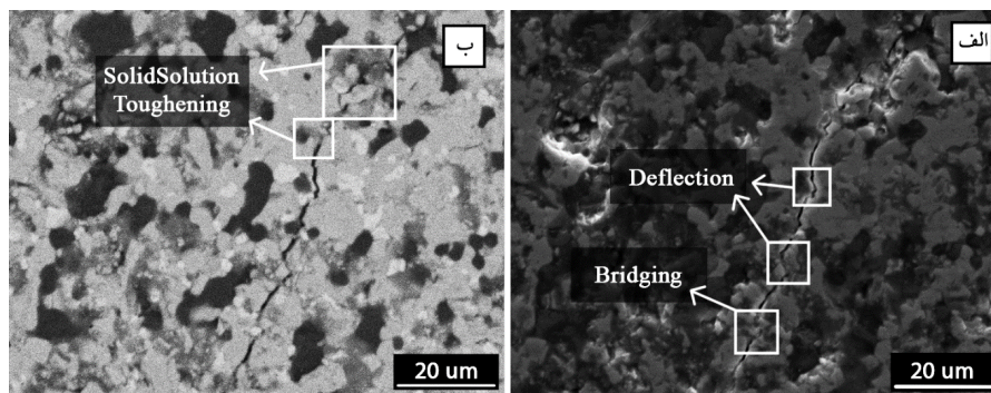
شکل ۱۰- تصویر SEM از مسیر رشد ترک در کامپوزیت \text{ZrB}_2\text{-}20 \text{ vol}\% \text{ SiC} - 15 \text{ vol}\% \text{ TiC} در مود الف (SE و ب) BSE.
