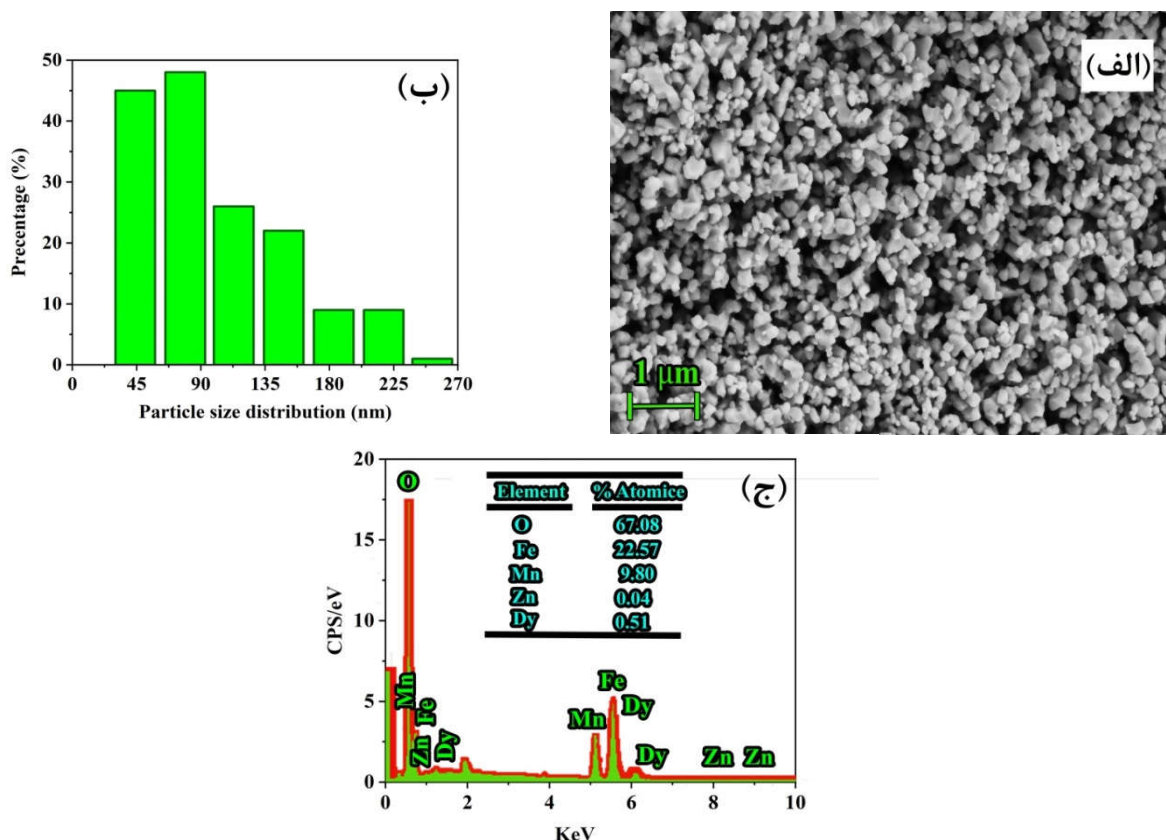
شکل ۳- (الف) تصویر FE-SEM نانوذرات تولیدشده، (ب) نمودار توزیع اندازه ذرات و (ج) نتایج حاصل از آنالیز EDS.
