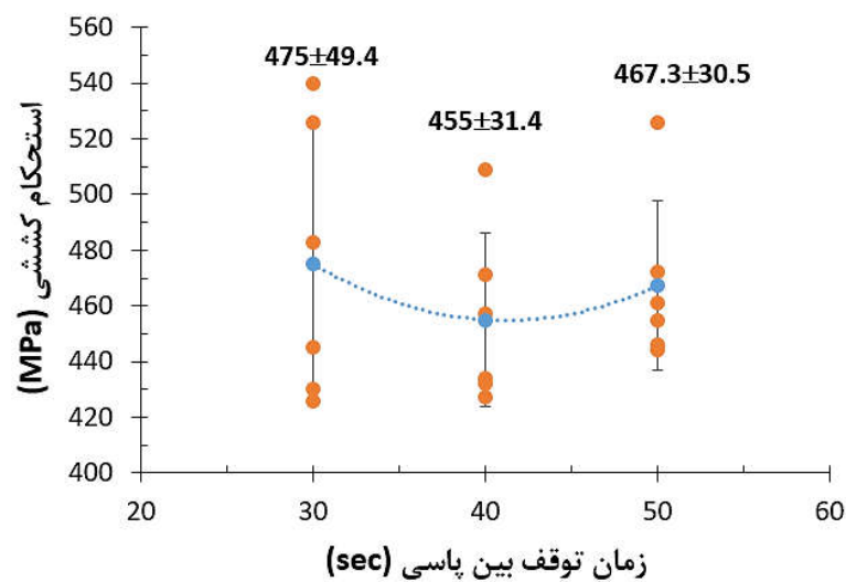
شکل ۱۰- ارتباط میان استحکام کششی با سرعت جوشکاری و زمان توقف بین پاسی.
