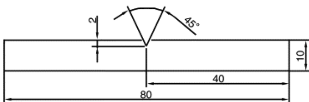
شکل ۳- نمونه استاندارد ISO 179 برای آزمون ضربه شارپی (۲۰).
