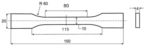
شکل ۲- ابعاد نمونه استاندارد ISO 527 (۱۹).
