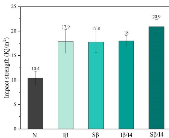
شکل ۸- استحکام ضربه نمونه‌ها.
