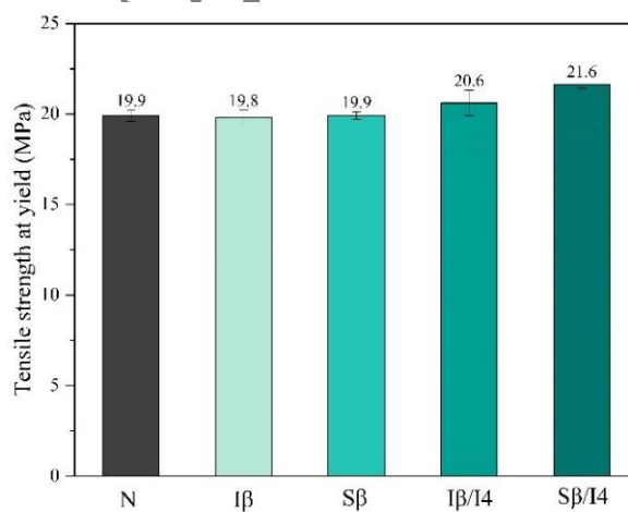
شکل ۶- تنش تسلیم نمونه‌ها.
