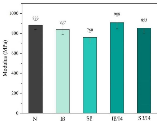
شکل ۷- مدول الاستیک نمونه‌ها.
