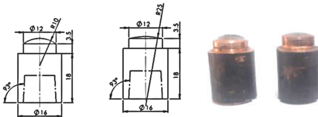
شکل ۵- هندسه الکتروودها.
