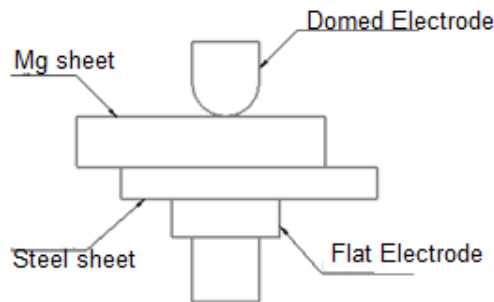
شکل ۳- شماتیک جوشکاری مقاومتی نقطه‌ای فولاد و منیزیم.
