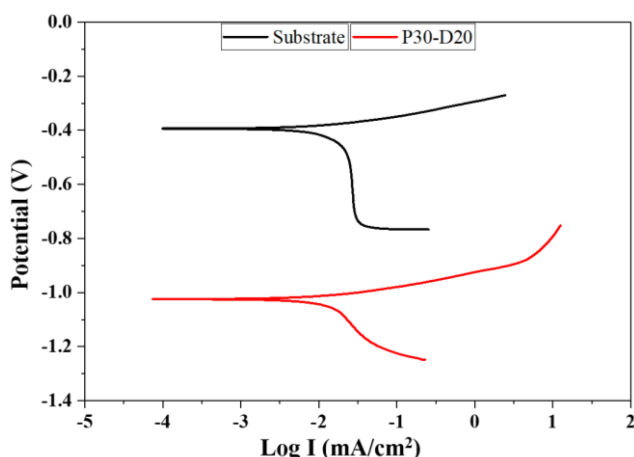
شکل ۷- نمودار پلاریزاسیون تافل پوشش روی و بستر فولادی در محلول ۳/۵ درصد نمک.
