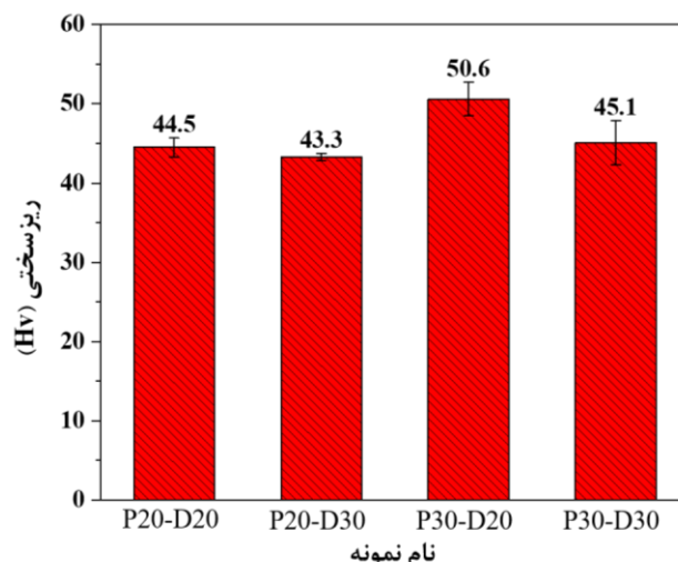
شکل ۸- ریزسختی پوشش‌های فلز روی در فشارهای ۲۰ و ۳۰ بار و فواصل پاشش ۲۰ و ۳۰ میلی‌متر (نمادهای P و D به ترتیب نشان‌دهنده فشار و فاصله پاشش هستند).
