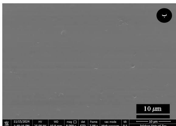
شکل ۷- تصاویر میکروسکوپی الکترونی روبشی گسیل میدانی سطح نمونه‌های (الف) آلومینا خالص، (ب) \text{Alumina+0.1\%wt Si}_3\text{N}_4\text{+2\%DI}
