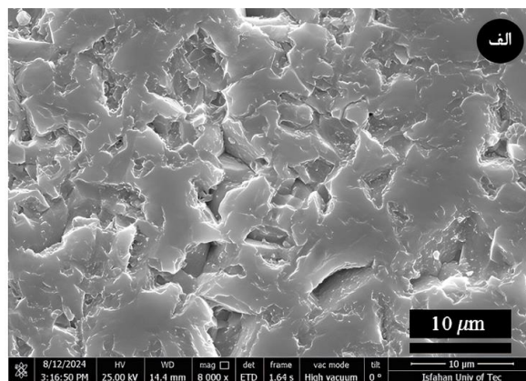
شکل ۷- تصاویر میکروسکوپی الکترونی روبشی گسیل میدانی سطح نمونه‌های
