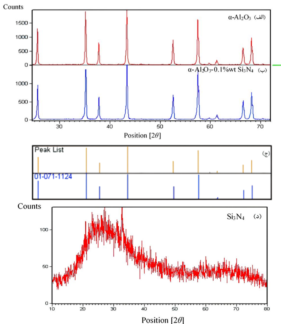
شکل ۳- آنالیز پراش پرتو ایکس نمونه‌های (الف) پودر آلومینا خالص، (ب) پودر کامپوزیت \alpha\text{-Al}_2\text{O}_3\text{-}0.1\%\text{Si}_3\text{N}_4 ، (ج) الگوی استاندارد، (د) پودر نیتريد سيليسيم.
