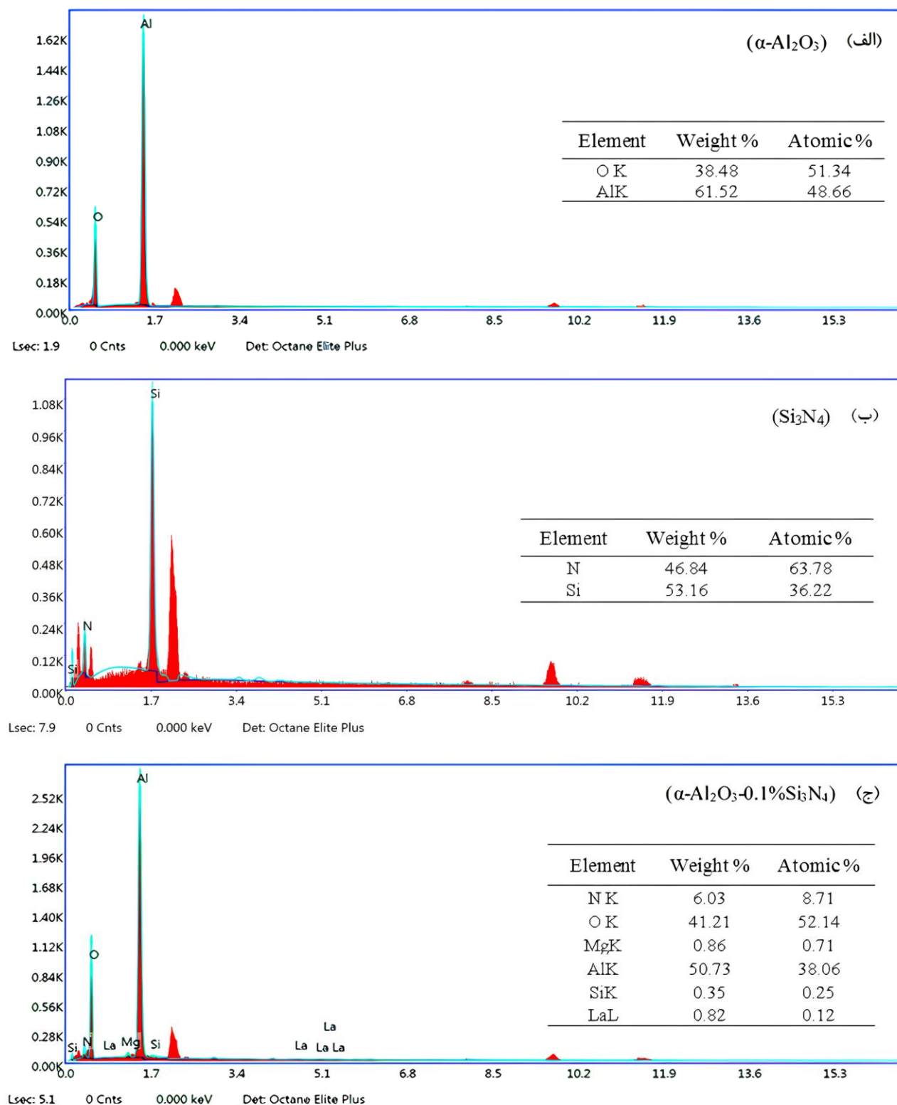
شکل ۴- آنالیز طیف سنجی تفکیک انرژی پرتو نمونه های
