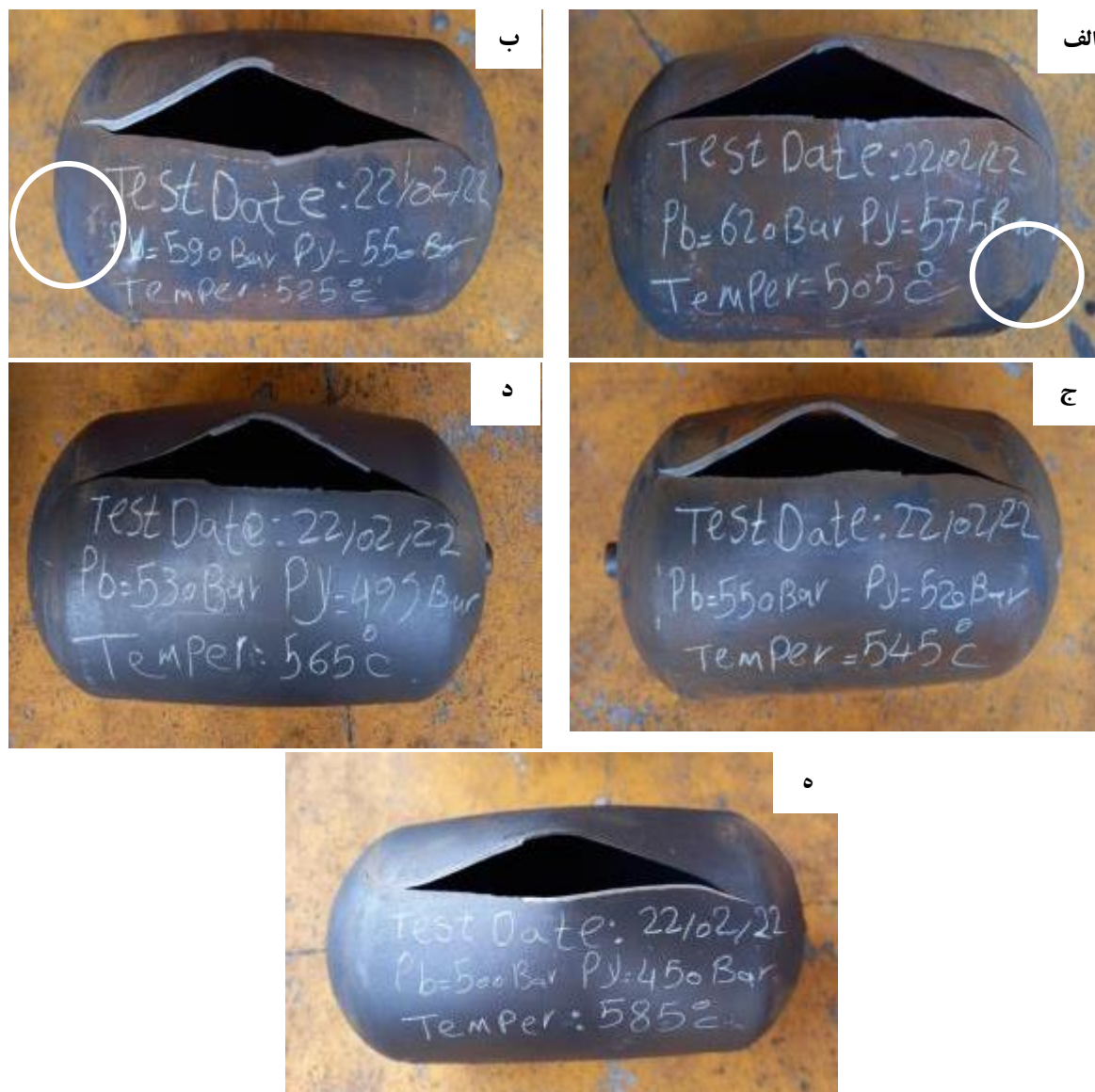
شکل ۱۱- تصاویر مخازن بازپخت شده در دماهای الف) ۵۰۵ °C، ب) ۵۲۵ °C، ج) ۵۴۵ °C، د) ۵۶۵ °C و ه) ۵۸۵ °C بعد از آزمون ترکیدن.
