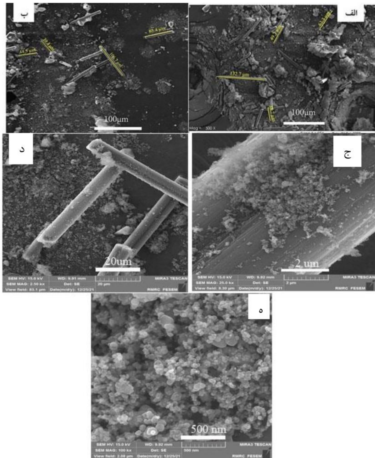
شکل ۸- تصاویر FESEM پودر کامپوزیتی MCMB-C/SiC با درصدی ریزدانه‌های مزوفاز کربنی:
