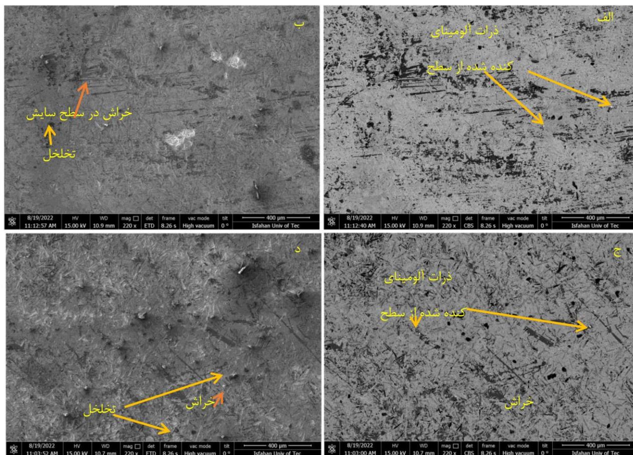
شکل ۱۳- تصاویر میکروسکوپی الکترونی روبشی گسیل میدانی در مد الکترون ثانویه و برگشتی از سطح سایش نمونه‌های MCMB-Cf/SiC تفجوشی‌شده به روش SPS: الف و ب) با ۱ درصد و ج و د) با ۱ درصد وزنی MCMB.
