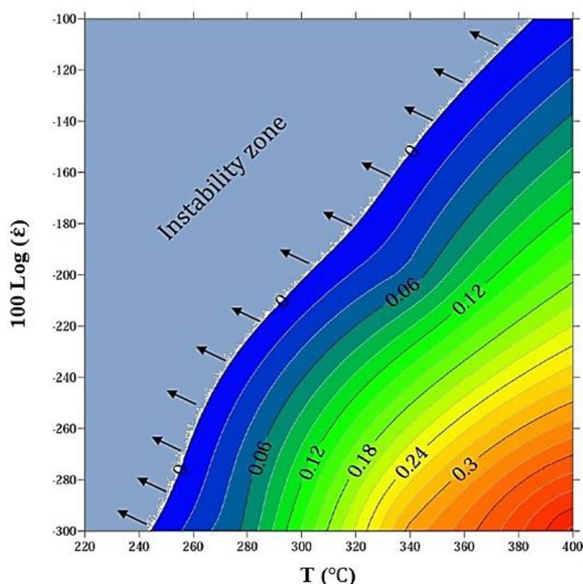
شکل ۹- نمودار نهایی نقشه فرایندی پارامتر \epsilon در کرنش ۰/۶.
