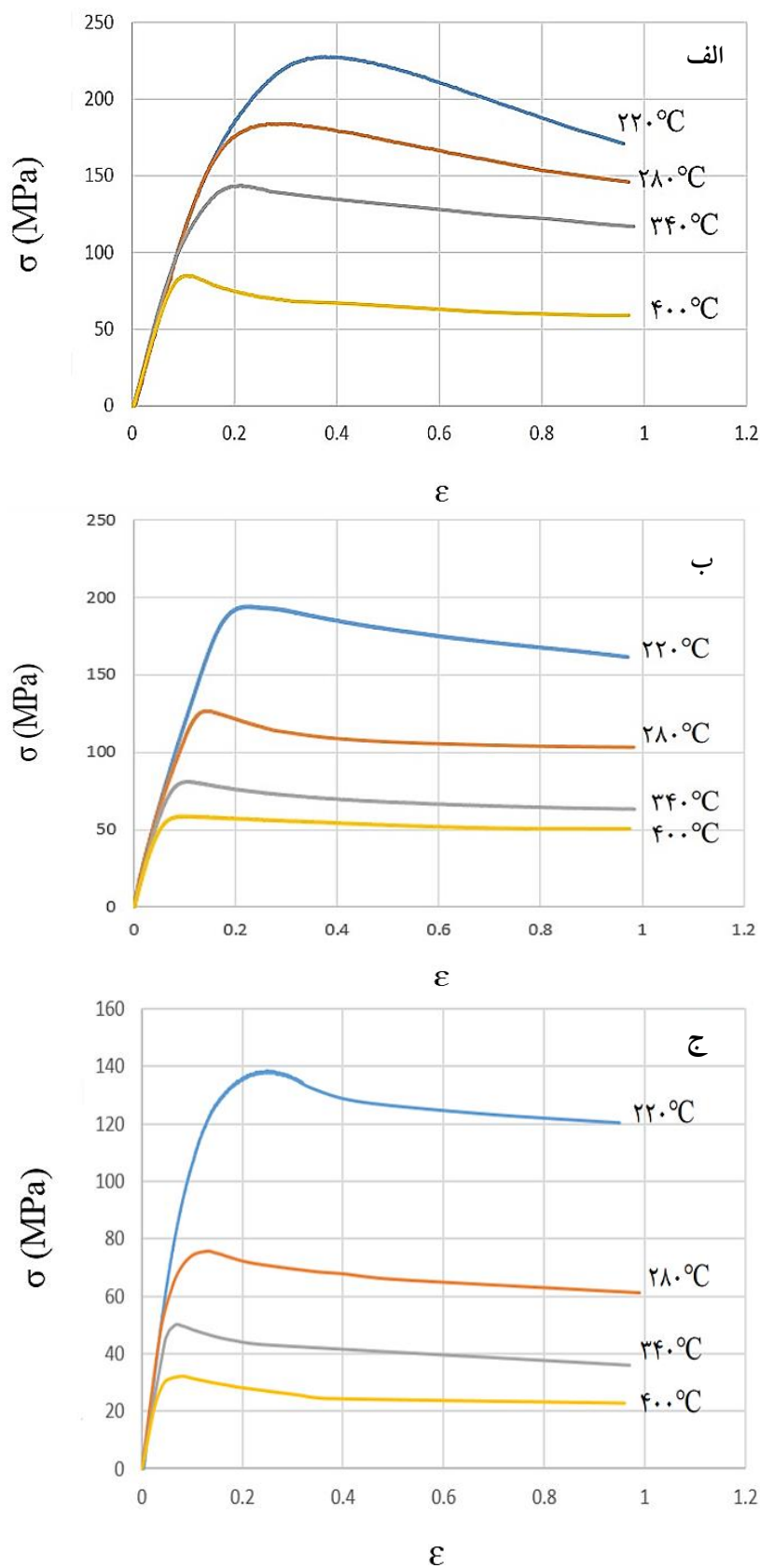
شکل ۳- نمودارهای تنش- کرنش در نرخ کرنش‌های (الف) ۱/۰، (ب) ۰/۰۱ و (ج) ۰/۰۰۱ بر ثانیه.
