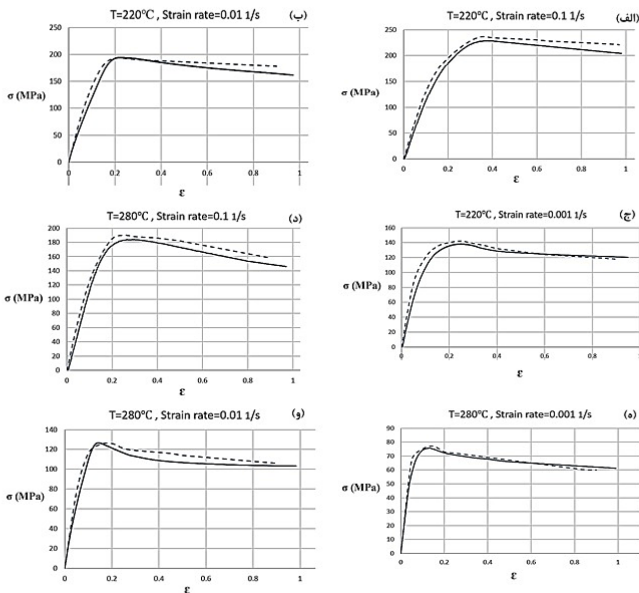
شکل ۵- مقایسه نمودار تنش- کرنش مدل آرنیوسی با حالت تجربی در دماهای ۲۲۰ و ۲۸۰ درجه سانتی گراد و نرخ کرنش‌های مختلف. خط کامل (—) نشان دهنده نمودار تنش- کرنش تجربی و خط چین (---) نشان دهنده نمودار تنش- کرنش مدل آرنیوسی در دما و نرخ کرنش: (الف) ۲۲۰ درجه سانتی گراد و ۰/۱ بر ثانیه (ب) ۲۲۰ درجه سانتی گراد و ۰/۰۱ بر ثانیه (ج) ۲۲۰ درجه سانتی گراد و ۰/۰۰۱ بر ثانیه (د) ۲۸۰ درجه سانتی گراد و ۰/۱ بر ثانیه (ه) ۲۸۰ درجه سانتی گراد و ۰/۰۱ بر ثانیه و (و) ۲۸۰ درجه سانتی گراد و ۰/۰۰۱ بر ثانیه.
