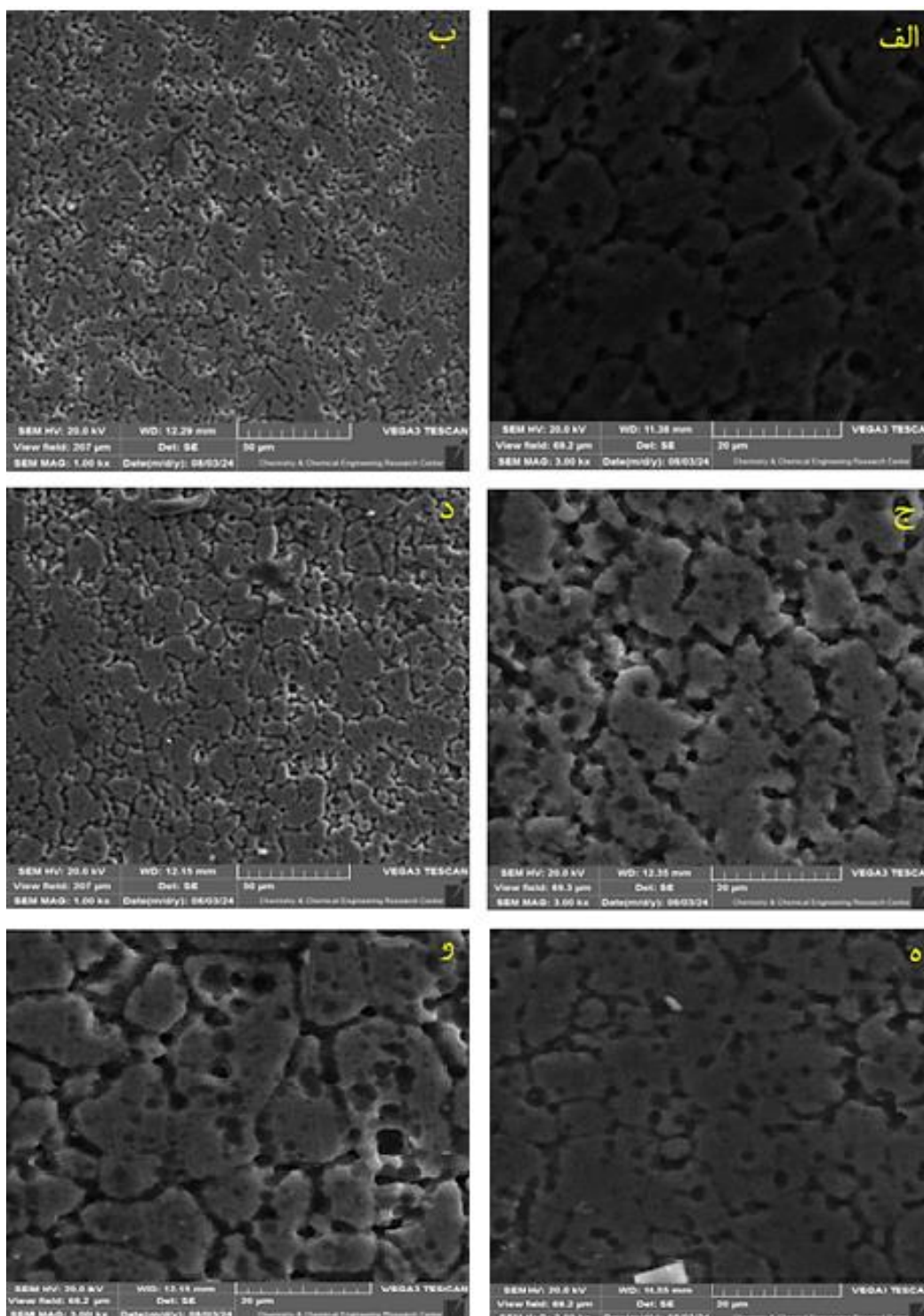
شکل ۱۱- تصاویر ریزساختاری آلیاژ Al-7.5Mg (سری دوم): الف) دما ۲۸۰ درجه سانتی‌گراد و نرخ کرنش ۱٪ بر ثانیه با بزرگنمایی ۳۰۰۰ در منطقه عدم تغییر شکل (ب) دما ۳۴۰ درجه سانتی‌گراد و نرخ کرنش ۱٪ بر ثانیه با بزرگنمایی ۱۰۰۰ (ج) دما ۳۴۰ درجه سانتی‌گراد و نرخ کرنش ۱٪ بر ثانیه با بزرگنمایی ۳۰۰۰ (د) دما ۳۴۰ درجه سانتی‌گراد و نرخ کرنش ۱٪ بر ثانیه با بزرگنمایی ۱۰۰۰ در منطقه عدم تغییر شکل (ه) دما ۴۰۰ درجه سانتی‌گراد و نرخ کرنش ۱٪ بر ثانیه با بزرگنمایی ۳۰۰۰ در منطقه عدم تغییر شکل (و) دما ۳۴۰ درجه سانتی‌گراد و نرخ کرنش ۱٪ بر ثانیه با بزرگنمایی ۳۰۰۰ برابر در منطقه عدم تغییر شکل.
