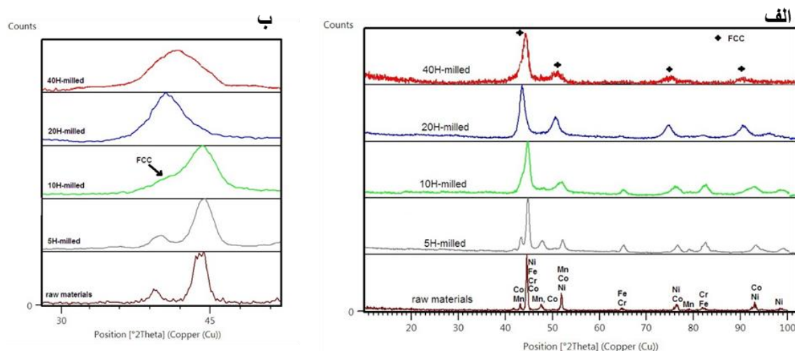
شکل ۲- تکامل فاز تابعی از زمان آلیاژسازی مکانیکی در آلیاژ انتروپی بالا FeCrCoNiMn (الف) و قسمت بزرگ‌شده شدیدترین قله الگوی XRD (ب).
