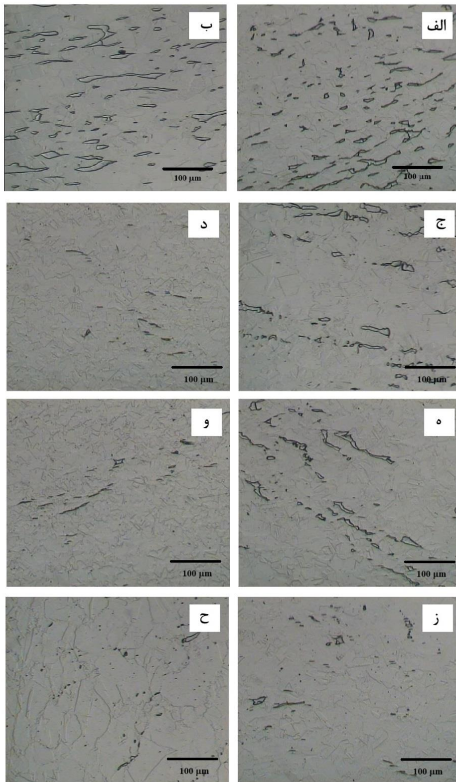
شکل ۳- تصاویر متالوگرافی مربوط به نمونه‌های (الف) ۳۰-۱۲۰۰، (ب) ۶۰-۱۲۰۰، (ج) ۳۰-۱۱۵۰، (د) ۶۰-۱۱۵۰، (ه) ۳۰-۱۱۰۰، (و) ۶۰-۱۱۰۰، (ز) ۳۰-۱۰۵۰ و (ح) ۶۰-۱۰۵۰.
