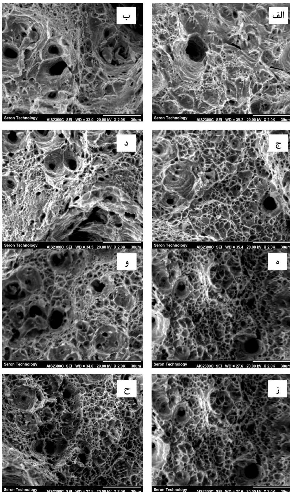
شکل ۷- تصویر شکست نگاری الف) نمونه ۳۰-۱۲۰۰، ب) نمونه ۶۰-۱۲۰۰، ج) نمونه ۳۰-۱۱۵۰، د) نمونه ۶۰-۱۱۵۰، ه) نمونه ۳۰-۱۱۰۰، و) نمونه ۶۰-۱۱۰۰، ز) نمونه ۳۰-۱۰۵۰ و ح) نمونه ۶۰-۱۰۵۰.
