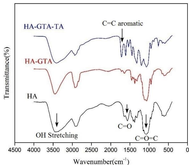
شکل ۲- نمودار طیف FTIR سه نمونه (HA)، (HA-GTA) و (HA-GTA-TA).
