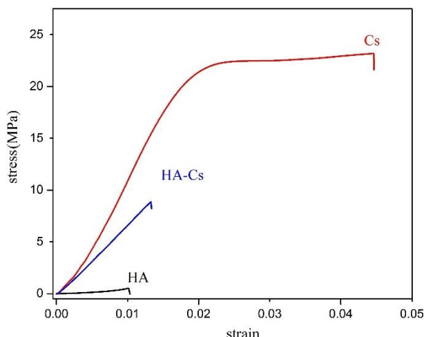
شکل ۵- نمودار تنش-کرنش فیلم‌های HA، HA-Cs و Cs.
