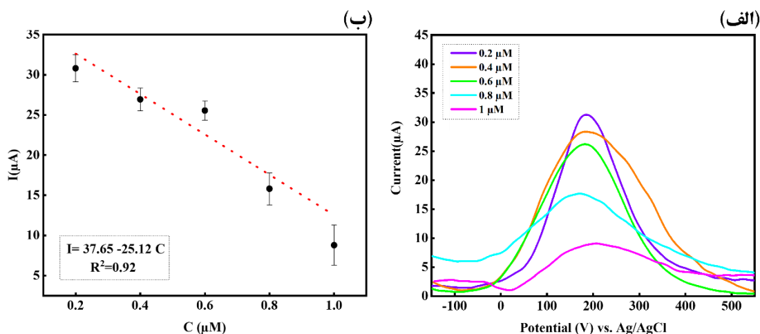
شکل ۶- الف) نتایج حاصل از آزمون ولتامتری پالس تفاضلی، ب) منحنی کالیبره نمونه MIP بر اساس جریان خروجی نسبت به غلظت‌های مختلف گلوکز در محدوده غلظت گلوکز ۱-۲٪ میکرومولار در محلول حاوی [Fe(CN)_6]^{3-} / [Fe(CN)_6]^{4-} .
