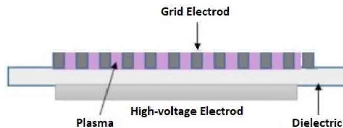
شکل ۱- طرحواره سامانه تولید پلاسمای سرد اتمسفری SDBD.
