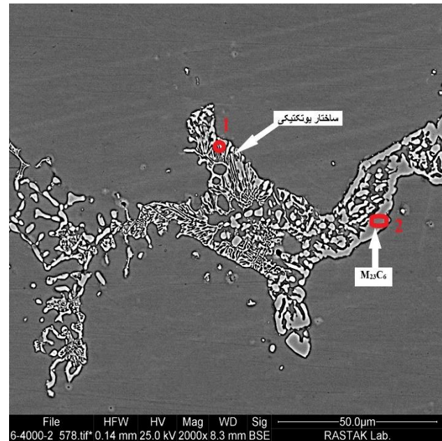
شکل ۱۰- ساختارهای یونکتیکی در سوپرآلیاژ پایه کبالت FSX-414.
