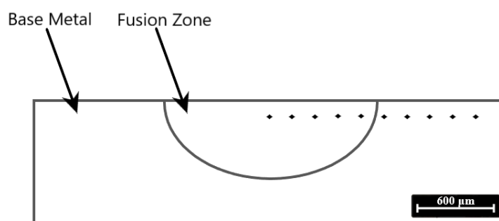
شکل ۵- طرح‌واره نحوه انجام آزمون ریزسختی سنجی.
