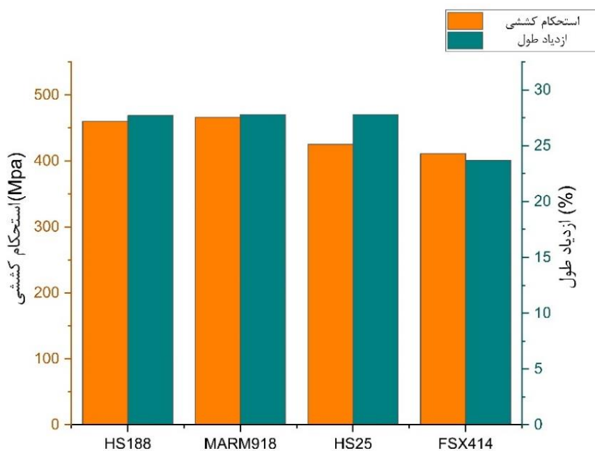
شکل ۲۹- نمودار میله‌ای مقایسه‌ای نتایج آزمون کشش در دمای بالا (۶۵۰ °C) برای نمونه‌های مختلف.
