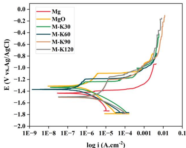
شکل ۶- نمودار تافل نمونه‌های پوشش داده شده با کراتین در زمان‌های مختلف.
