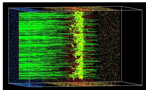
شکل ۱- نمایش طرحواره هندسه در شبیه‌ساز Geant4.
