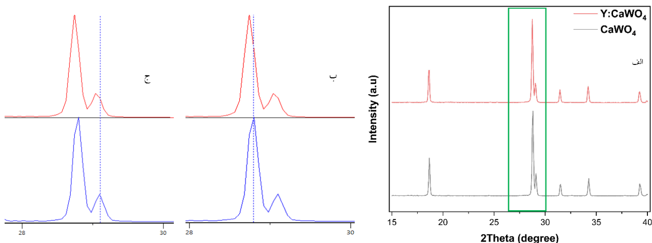
شکل ۳- الف) الگوی تفرق اشعه ایکس تنگستات کلسیم و تنگستات کلسیم آلاینده شده با ایتريوم سنتز شده با روش هم‌رسوبی بعد از عملیات کلسینه، ب) و ج) مقایسه دو الگو با بزرگنمایی بالاتر برای بررسی جابجایی پیک‌ها.
