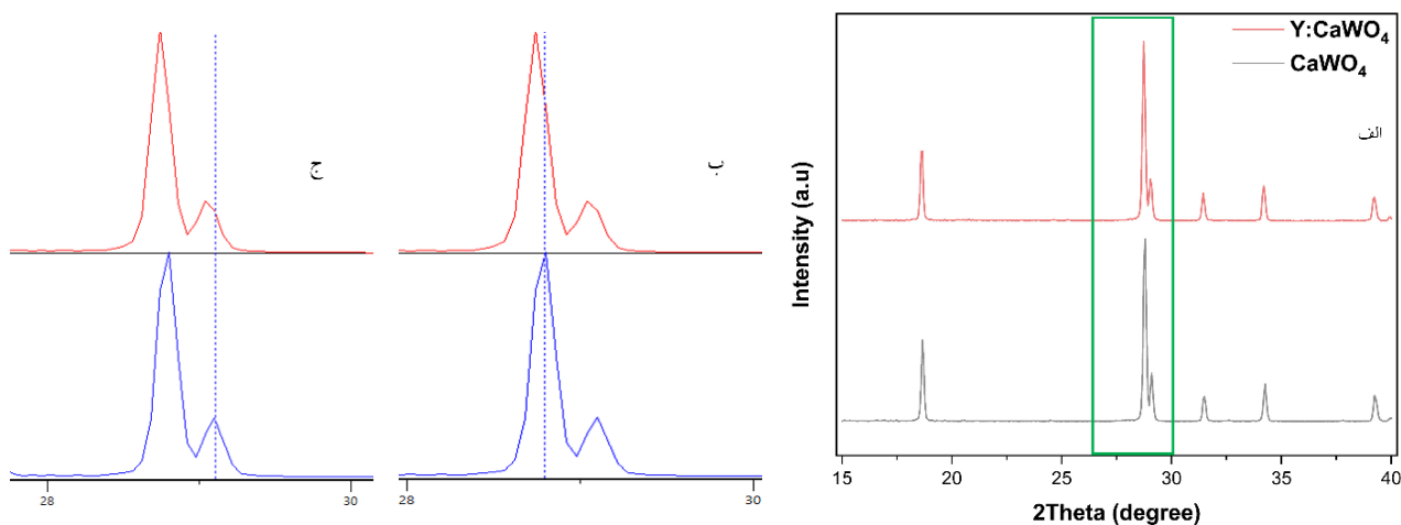
شکل ۳- الف) الگوی تفرق اشعه ایکس تنگستات کلسیم و تنگستات کلسیم آلائیده شده با ایتريوم سنتز شده با روش هم‌رسویی بعد از عملیات کلسینه، ب) و ج) مقایسه دو الگو با بزرگنمایی بالاتر برای بررسی جابجایی پیک‌ها.
