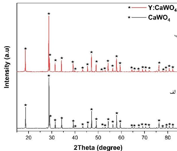
شکل ۲- الگوی تفرق اشعه ایکس: الف) تنگستات کلسیم، ب) تنگستات کلسیم آلائیده شده با ایتريوم با روش هم‌رسویی بعد از عملیات کلسینه‌شدن.
