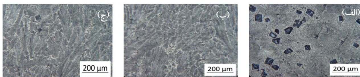
شکل ۴- تصاویر ریزساختار آلیاژ یوتکتیک ذوب مجدد شده Al-13.8%Mg 2 Si ریخته‌گری شده به روش ثقلی حاوی جوانه‌زای Al-5Zr در
