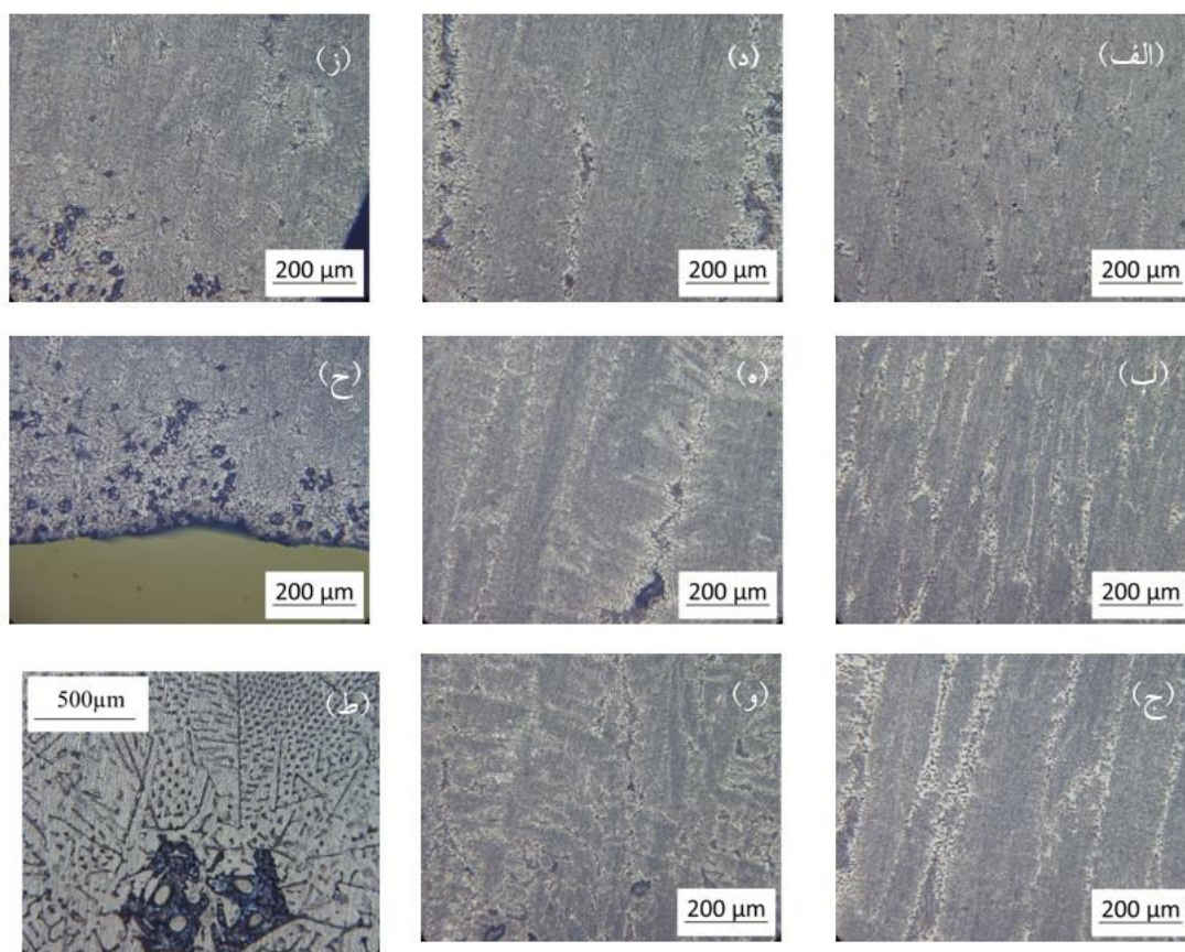
شکل ۸- تصاویر ریزساختار میکروسکوپی نوری آلیاژ Al-13.8%Mg 2 Si حاوی ۰/۱ درصد وزنی جوانه‌زای Al-5Zr پس از ریخته‌گری گریز از مرکز (از (الف) تا (ح)، به ترتیب دلالت دارند بر ریزساختار خارجی‌ترین سطح استوانه ریختگی تا داخلی‌ترین سطح آن)، (ط) ریزساختار داخلی‌ترین لایه.
