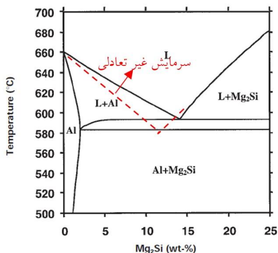
شکل ۵- تغییر موقعیت نقطه یوتکتیک در نمودار فازي تعادلي Al-Mg 2 Si در اثر انجماد غیر تعادلي (۲۲).
