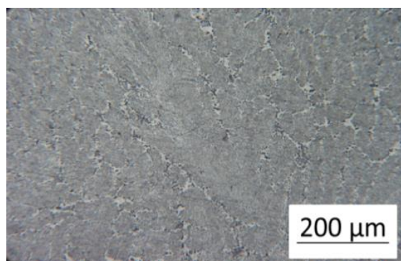
شکل ۲- ریزساختار شمش ذوب مجددشده با ترکیب یوتکتیک
