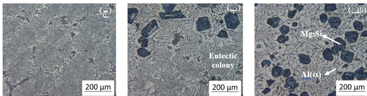
شکل ۳- تصاویر ریزساختارهای آلیاژ یوتکتیک Al-13.8%Mg 2 Si ریخته‌گری شده به روش ثقلی بدون جوانه‌زا
