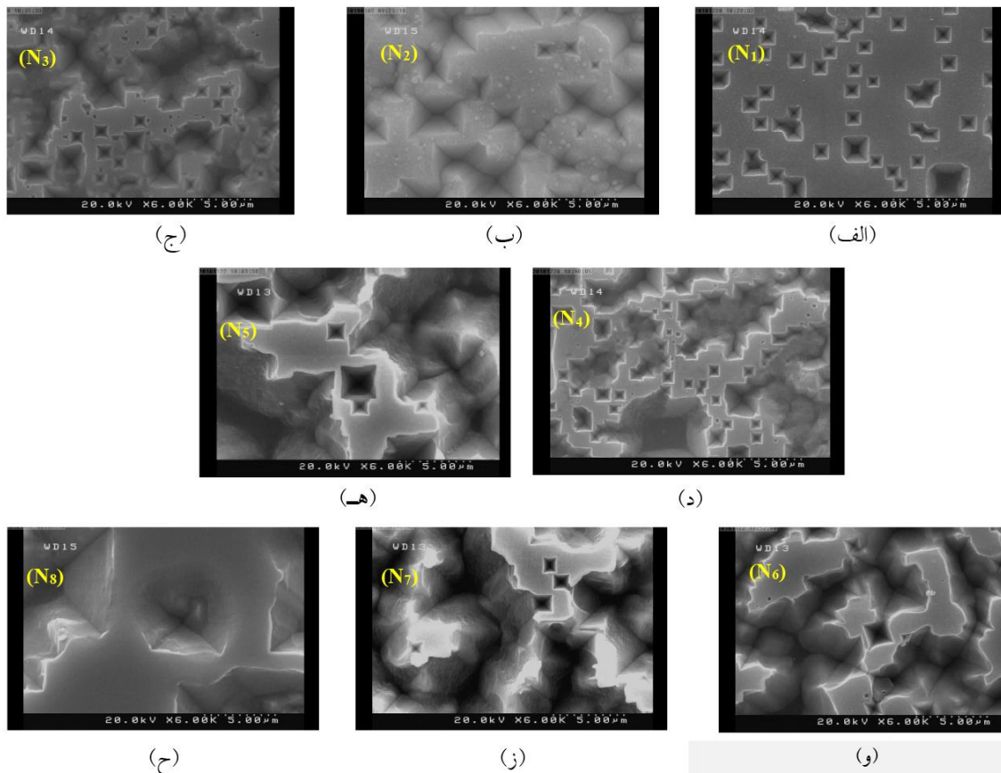
شکل ۶- ساختارهای شکل گرفته بر بستر سیلیکونی در محلول نیترات مس ۰/۰۵ مولار و هیدروفلوئوریک اسید ۴/۶ مولار در دمای ۵۰ درجه سانتی گراد و بدون پس زدایش در زمان‌های: (الف) ۱۰ ثانیه، (ب) ۲۰ ثانیه، (ج) ۳۰ ثانیه، (د) ۱ دقیقه، (ه) ۲ دقیقه، (و) ۳ دقیقه، (ز) ۴ دقیقه و (ح) ۵ دقیقه
