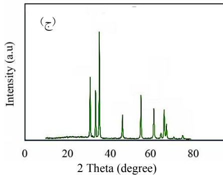
شکل ۴- الگوی پراش پرتو ایکس نمونه S75 سنتز شده در دمای کلسینه:
