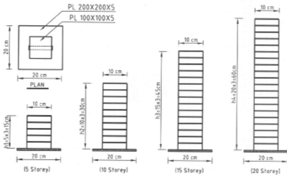
شکل ۸- مشخصات مدل‌های سازه ای ۲۰، ۱۵، ۱۰، ۵ و ۲۰ طبقه
