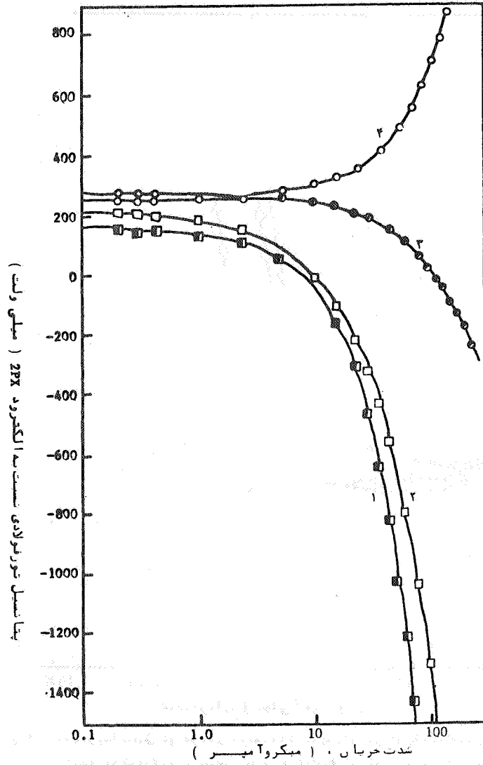
شکل ۴ تغییر پتانسیل تور فولادی بعنوان تابعی از شدت جریان برای پلاریزاسیون کاتدی صفحه فولادی . منحنی‌های ۴۰۳،۲۰۱ بر ترتیب پتانسیل تور فولادی در موقعیت ۴۰۳،۲۰۱ نسبت به الکتروود 2Pb در موقعیت ۴ را نشان میدهد .
