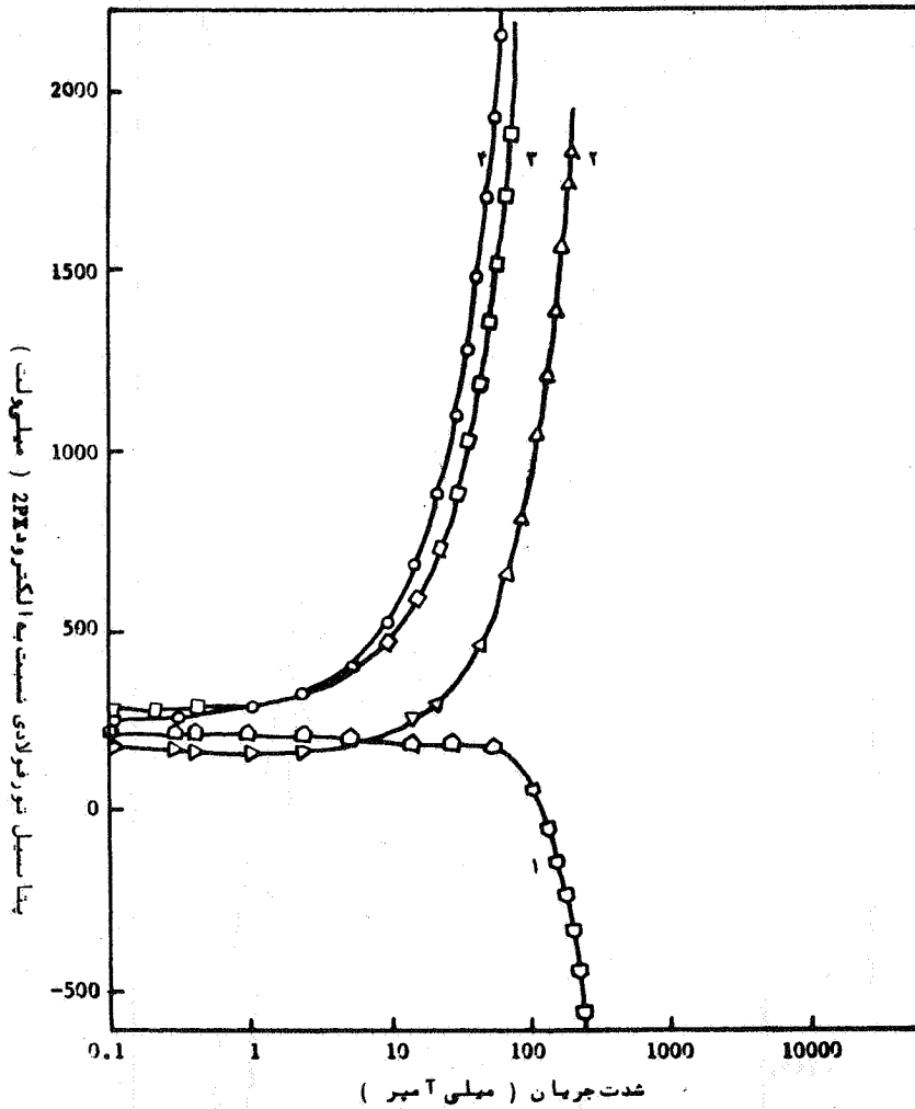
شکل ۷ - تغییر پتانسیل تور فولادی نسبت به شدت جریان برای پلاریزاسیون کاتدی صفحه فولادی. منحنی های ۱، ۲ و ۳ به ترتیب پتانسیل تور فولادی در موقعیت ۲، نسبت به الکتروود 2PXD در موقعیت ۲ را نشان می دهد.
