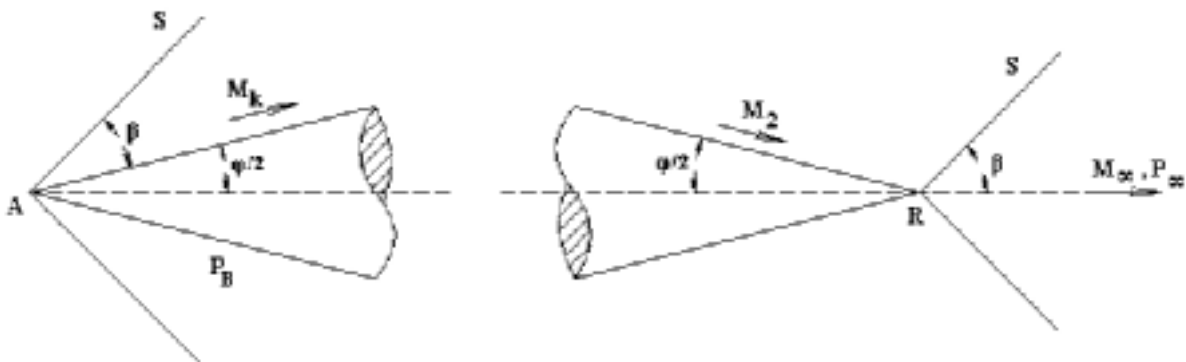
شکل ۵- تشابه سازی جریان مخروطی بادنباله
