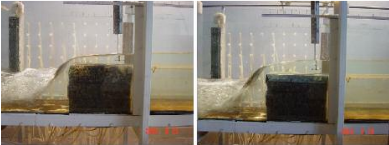
شکل ۳ - سمت چپ تاج نفوذپذیر و سمت راست تاج نفوذ ناپذیر
