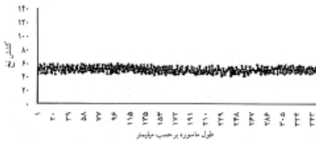
شکل ۷- تغییرات کشتش نخ از ابتدا تا انتهای ماسوره همراه با سیستم کنترل
