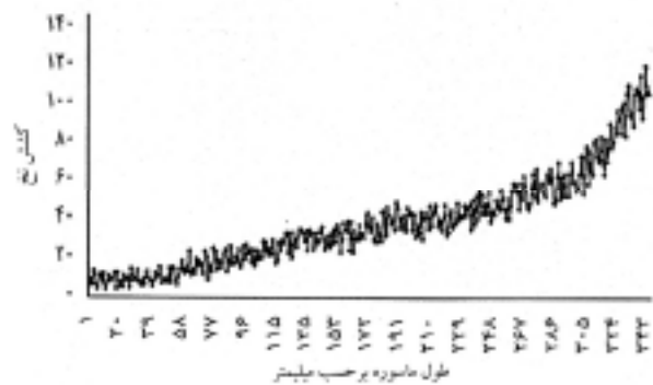
شکل ۶- تغییرات کشتش نخ از ابتدا تا انتهای ماسوره بدون سیستم کنترل
