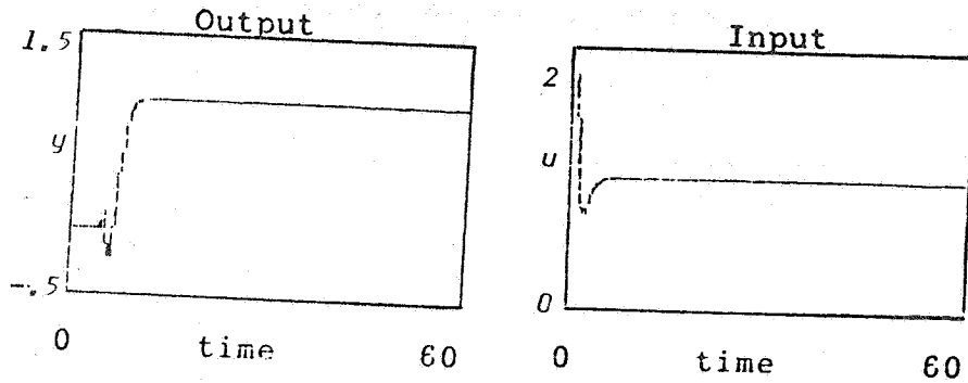
شکل ۱۸- پاسخ نسبت به تغییر پله‌ای واحد در y_T برای کنترل کننده‌های IMC ، مدار پیس خور معادل IMC و MBC ، بدون محدودیت در ورودی (مثال ۲)
