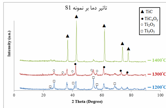
شکل ۱۰- الگوی پراش نمونه‌ی S1 را در دماهای 1200^\circ C ، 1300^\circ C و 1400^\circ C
