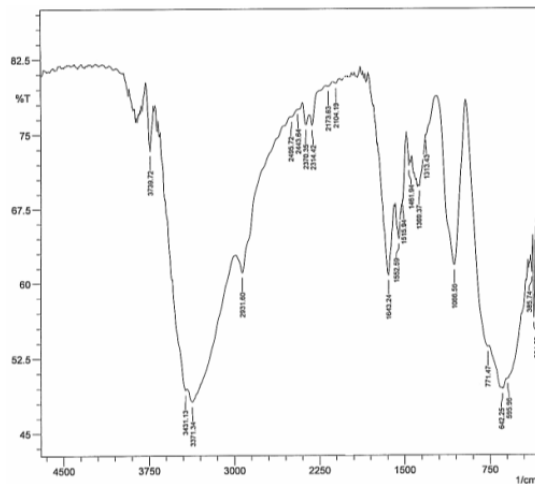
شکل ۴- طیف FTIR برای ژل خشک شده‌ی S1 در دمای 110^{\circ}\text{C} به مدت ۲۴ ساعت
