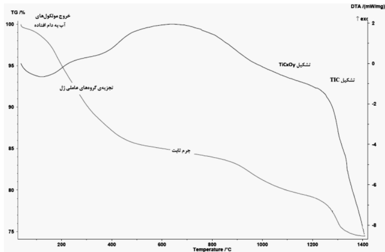
شکل ۶- منحنی DTA-TG برای نمونه‌ی S1
