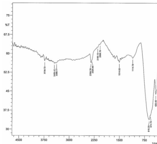
شکل ۵- طیف FTIR برای پودر S1 پخت شده در دمای 1400^{\circ}\text{C} به مدت یک ساعت
