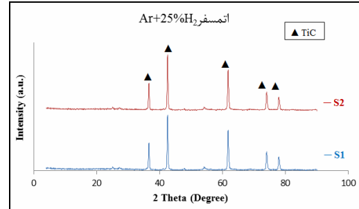
شکل ۹- الگوی پراش نمونه‌های S1 و S2 کلسینه شده در اتمسفر Ar+25\%H_2 در دمای 1400^\circ C به مدت یک ساعت
