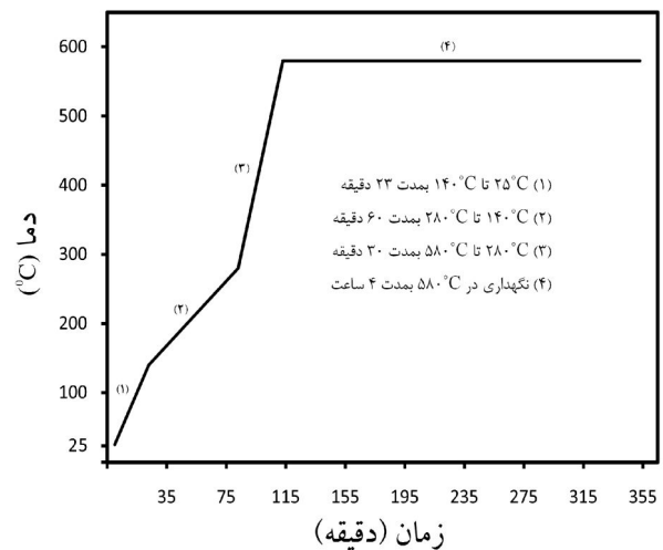
شکل ۴- سیکل عملیات خروج کربامید و زیتتر شدن نمونه‌ها
