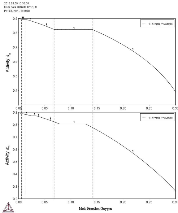
شکل ۳- منحنی‌های اکتیویته تیتانیوم در دماهای: الف) ۱۲۰۰، ب) ۱۷۰۰، ج) ۱۹۶۰ کلوین مربوط به این تحقیق در پایین و تحقیق همپل در بالای شکل
