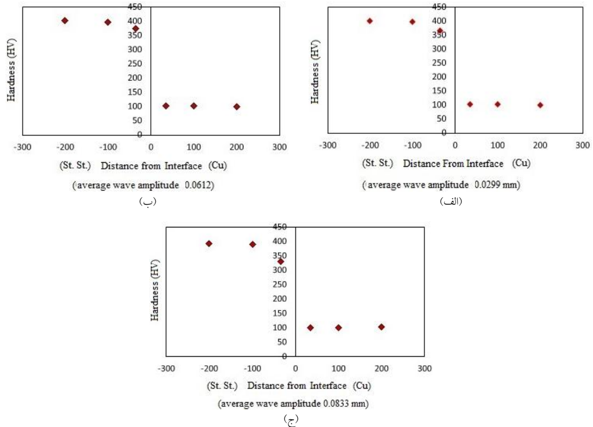
شکل ۱۴- پروفیل ریز سختی در نزدیک فصل مشترک اتصالات: الف) آزمون یک، ب) آزمون دو، ج) آزمون سه
