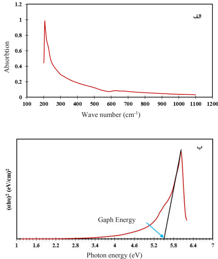
شکل ۶- الف) طیف نوری جذبی ثبت شده با طیف‌سنجی ماوراء بنفش- مرئی و ب) نمودار انرژی فوتون
