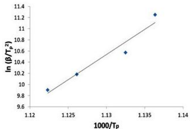
شکل ۲۵- نمودار آرنیوس مربوط به استحاله تبلور مرحله اول در آلیاژ Fe_{51}Cr_{18}Mo_7B_{16}C_4Nb_5
