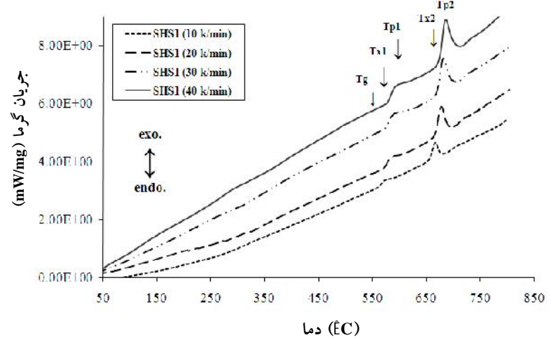
شکل ۳- نمودار DSC آلیاژ Fe 55 Cr 18 Mo 7 B 16 C 4 (SHS1)
