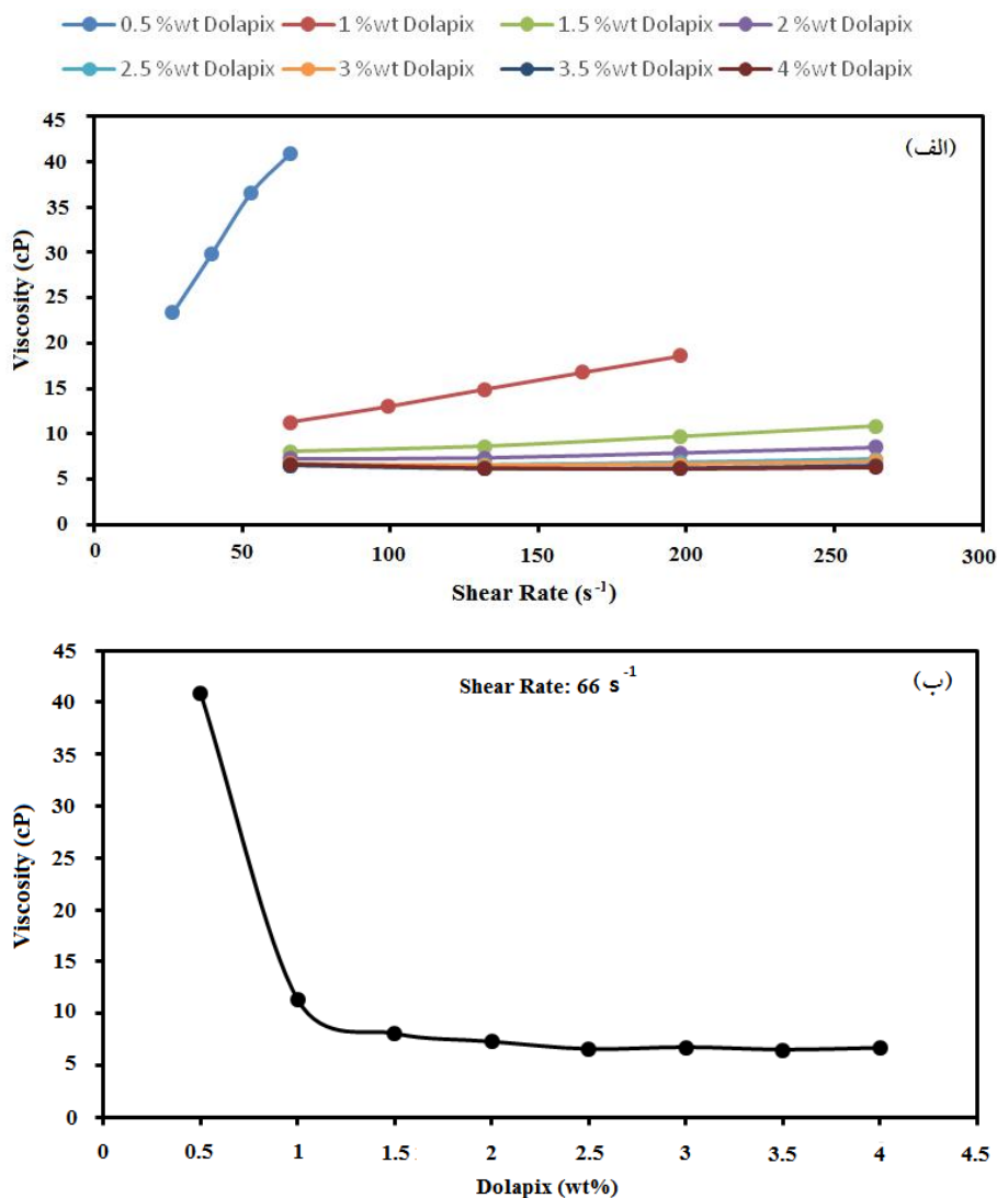
شکل ۴- الف) نمودار گرانروی - نرخ برشی دوغاب پودر نانوکامپوزیتی آلومینا/ ایتریا به عنوان تابعی از مقدار پراکنده ساز دولاپیکس در اسیدیته 10^{\circ} ، ب) روند تغییر گرانروی دوغاب با تغییر غلظت دولاپیکس
