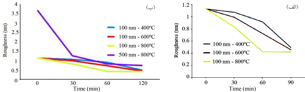
شکل ۳- مقایسه زبری فیلم سیلیسیم آنیل شده در دماهای مختلف: الف) ضخامت ۱۰۰ نانومتر و ب) ۱۰۰ و ۵۰۰ نانومتر (رنگی در نسخه الکترونیکی)
