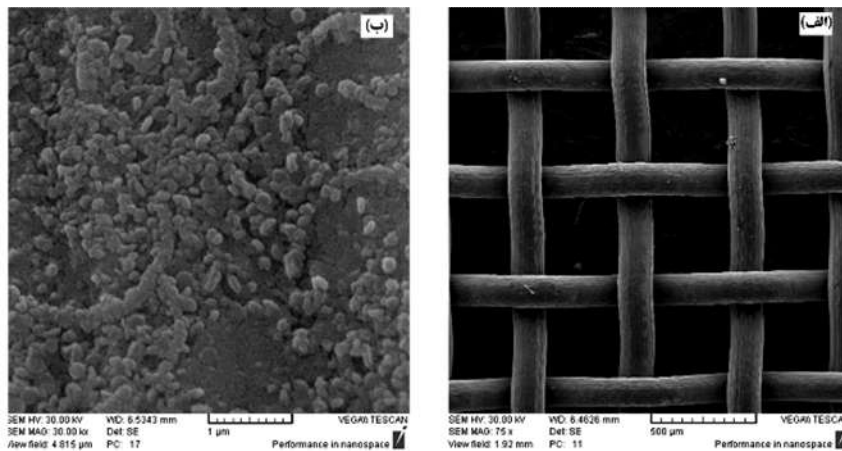
شکل ۱- تصاویر میکروسکوپی الکترونی روبشی از سطح توری استیل: الف) توری خام و ب) بعد از ایجاد بذر لایه
